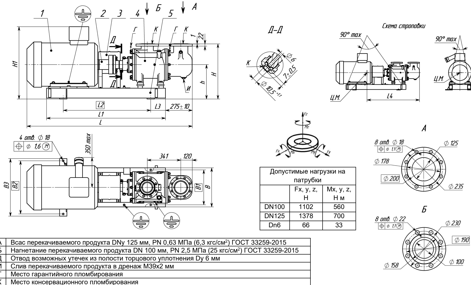
Рисунок Б.2 – Габаритный чертеж агрегата 1 – электродвигатель; 2 – муфта; 3 – кожух защитный; 4 – насос А2 3В 63/25Б; 5 – рама
