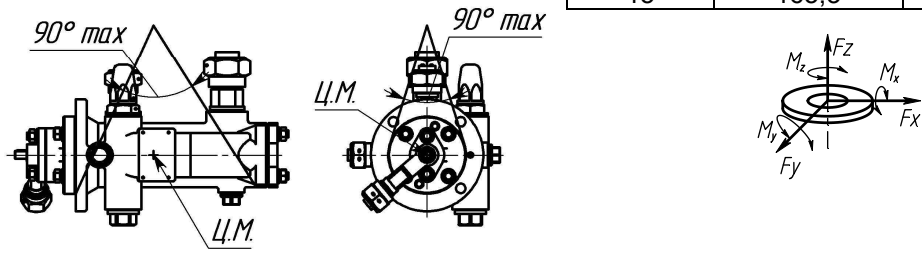
Схема строповки
