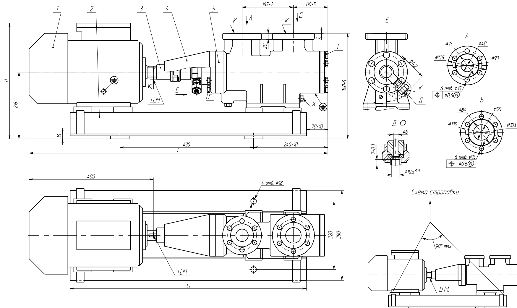
Рисунок Б.2 – Габаритный чертёж агрегата типа А4 3В 1,6/40
