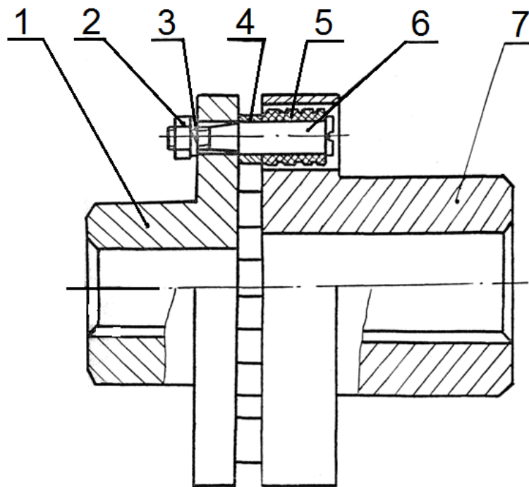
Рисунок 4 - Муфта
