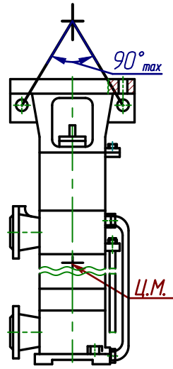
Схема строповки
