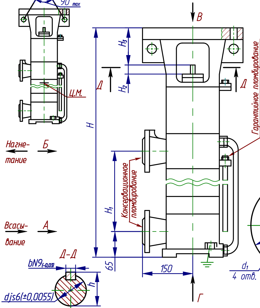
Приложение Б (обязательное) Габаритный чертеж насоса ЦНСв
