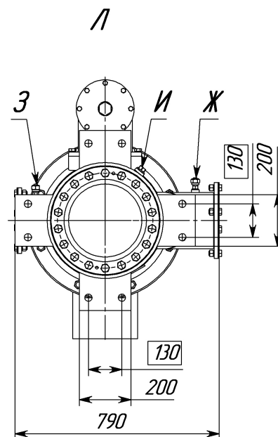
Схема строповки
