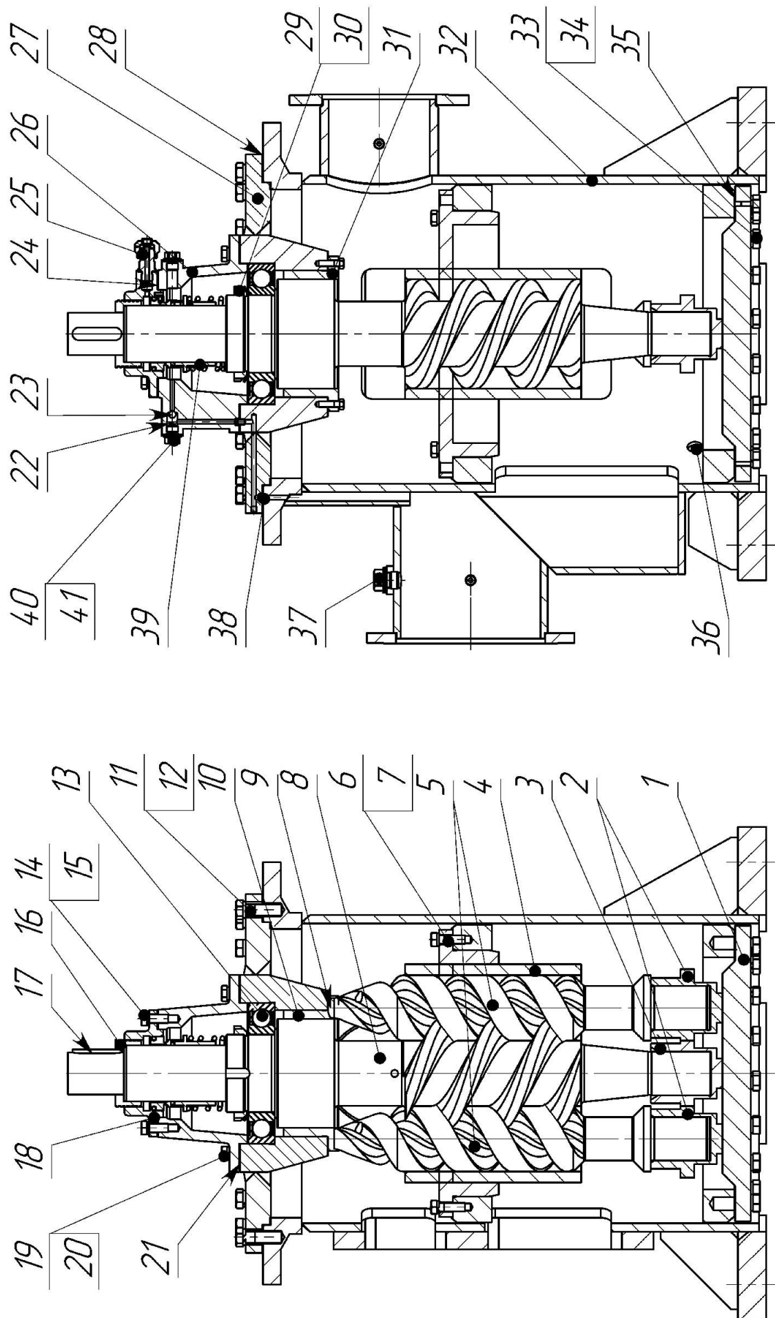
Рисунок 1 – Устройство насоса
