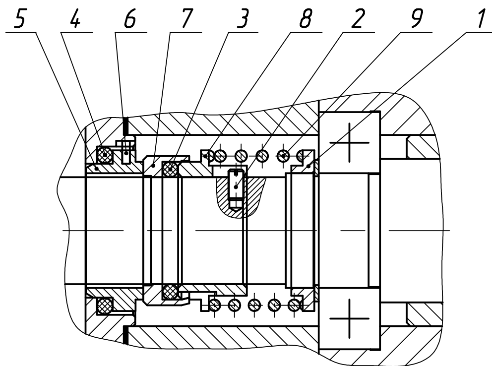
Рисунок 4 – Торцовое уплотнение
