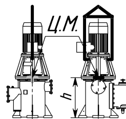
Схема строповки
