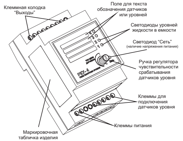
Рисунок 1 - Внешний вид
