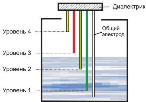
Рисунок 2 - Неметаллическая емкость
