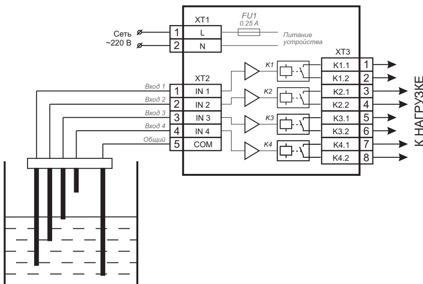
FU1 - предохранитель внутри корпуса устройства 0,25 А 250 В
