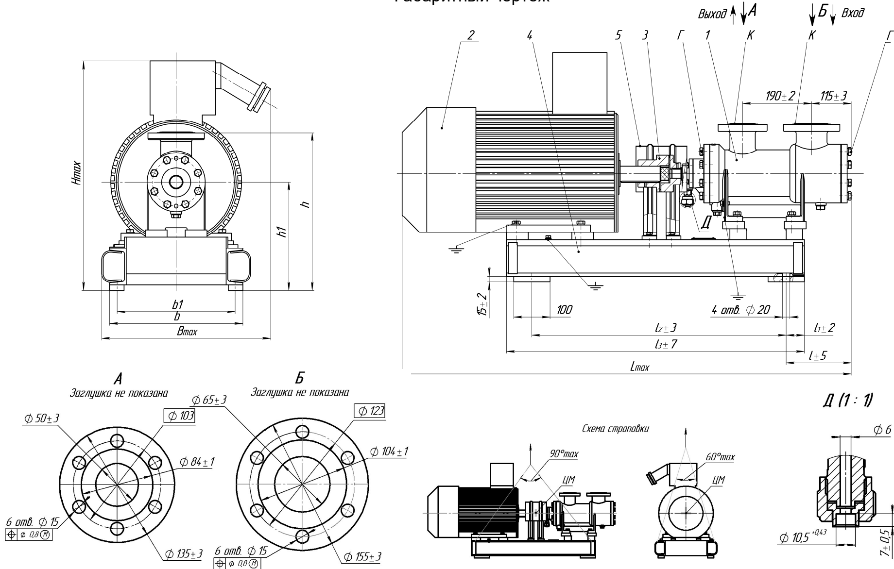
Рисунок Б1- Габаритный чертеж агрегатов электронасосных на базе насоса А5 3В 8/25
