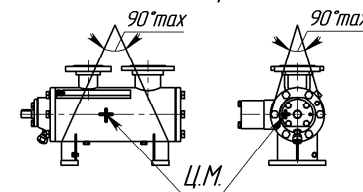
Схема строповки
