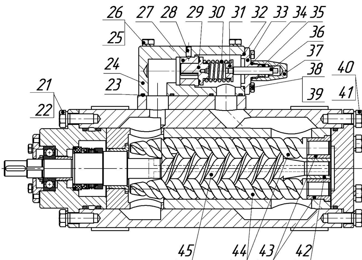
Рисунок 1 – Устройство насоса
