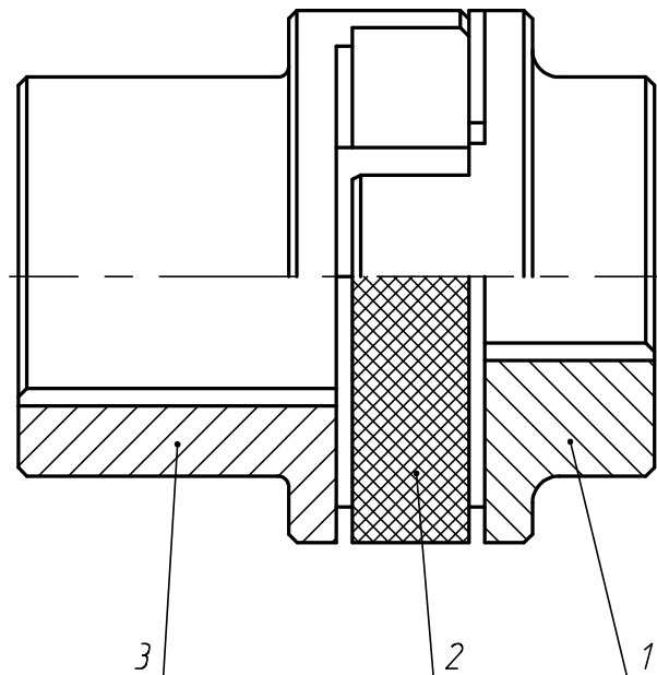
Рисунок 2 - Муфта
