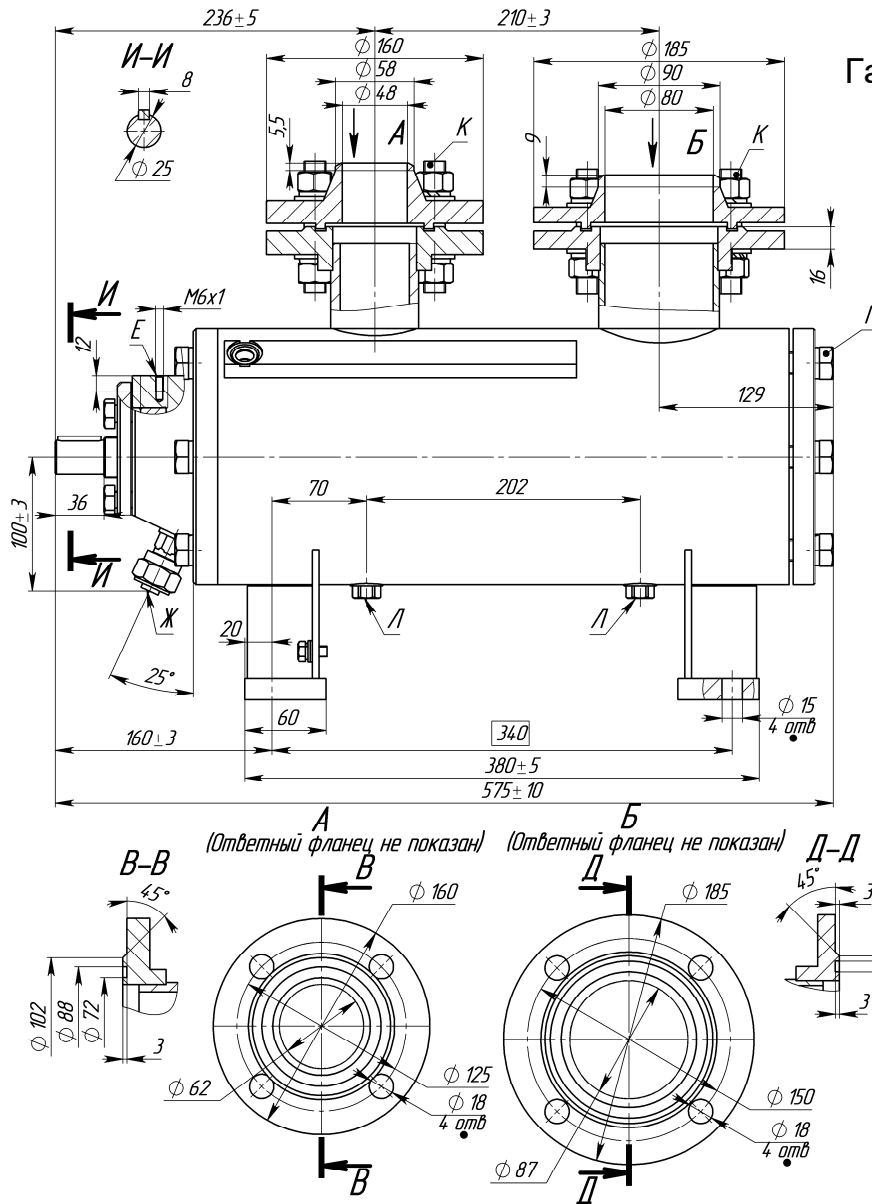
Рисунок Б.1 - Габаритный чертеж насоса А1 3В 8/40, А1 3В 10/35, А1 3В 12/25
