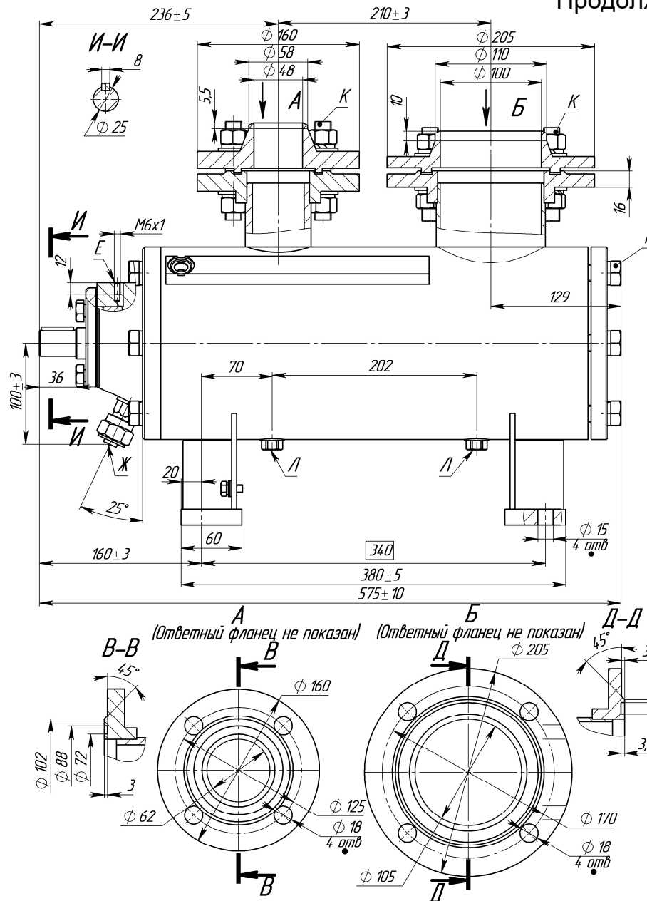
Рисунок Б.2 - Габаритный чертеж насоса АЗ 3В 16/25
