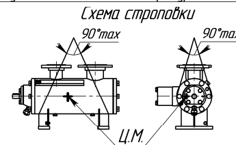
Рисунок Б.1 - Габаритный чертеж насоса А1 3В 8/40, А1 3В 10/35, А1 3В 12/25
