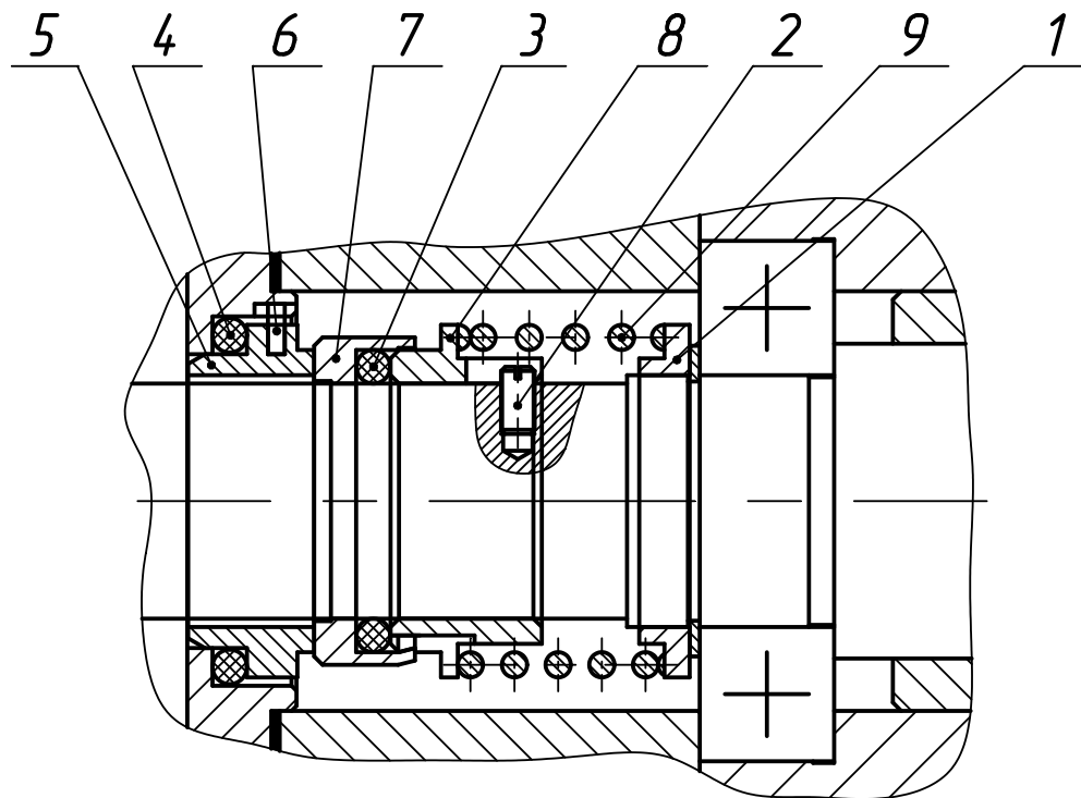
Рисунок 4 – Торцовое уплотнение
