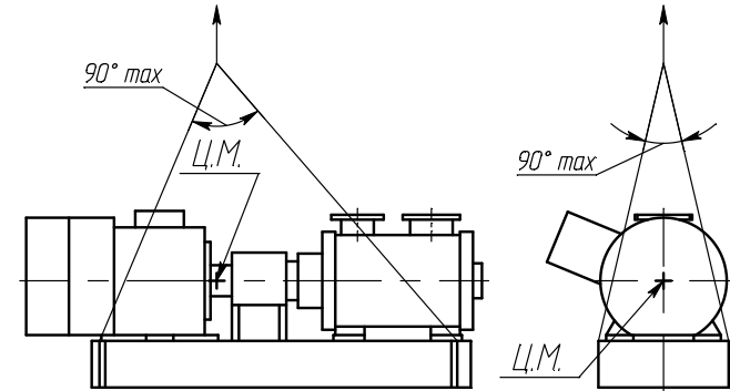
Схема строповки
