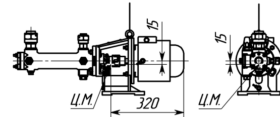
Схема строповки
