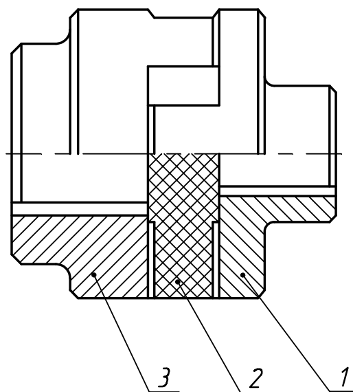
Рисунок 3 – Муфта
