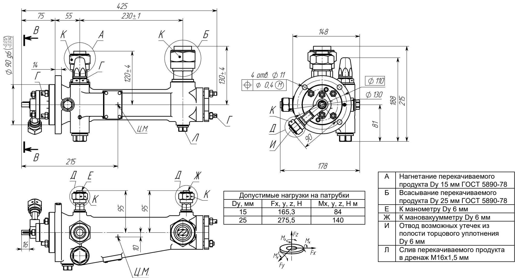
Рисунок Б.2 – Габаритный чертеж насоса А1 3В 0,6/63
