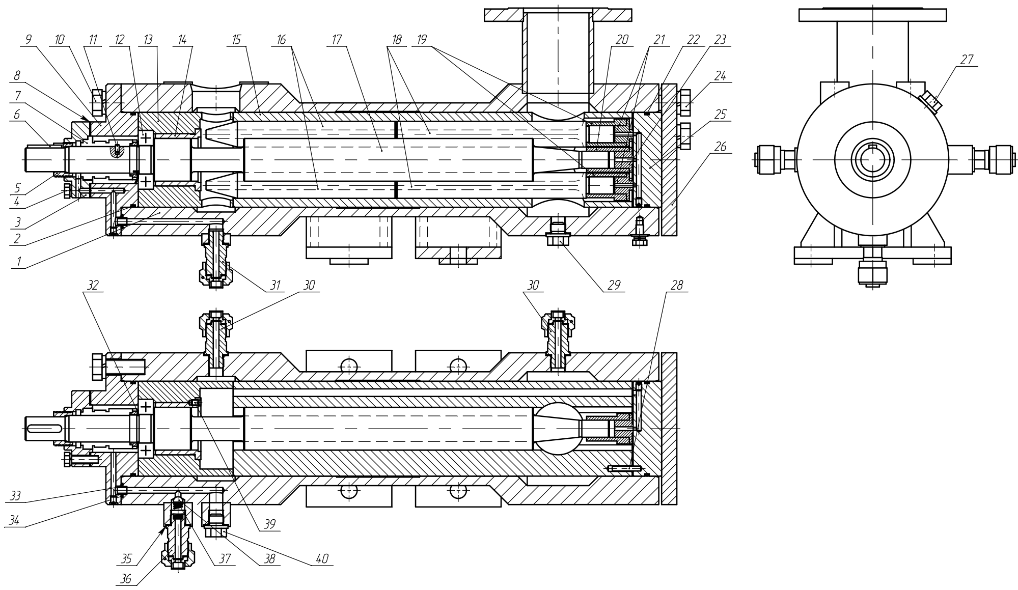
Рисунок 1 – Устройство насоса
