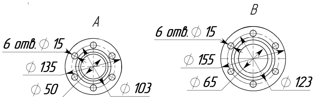
Нагнетание Ду50 Ру25 ГОСТ 1536-76
