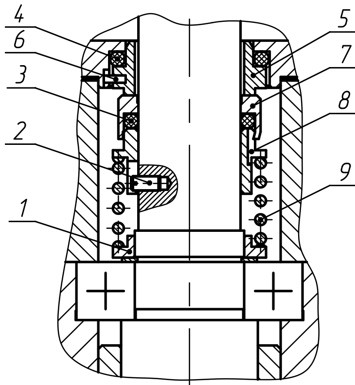
Рисунок 4 – Уплотнение торцовое
