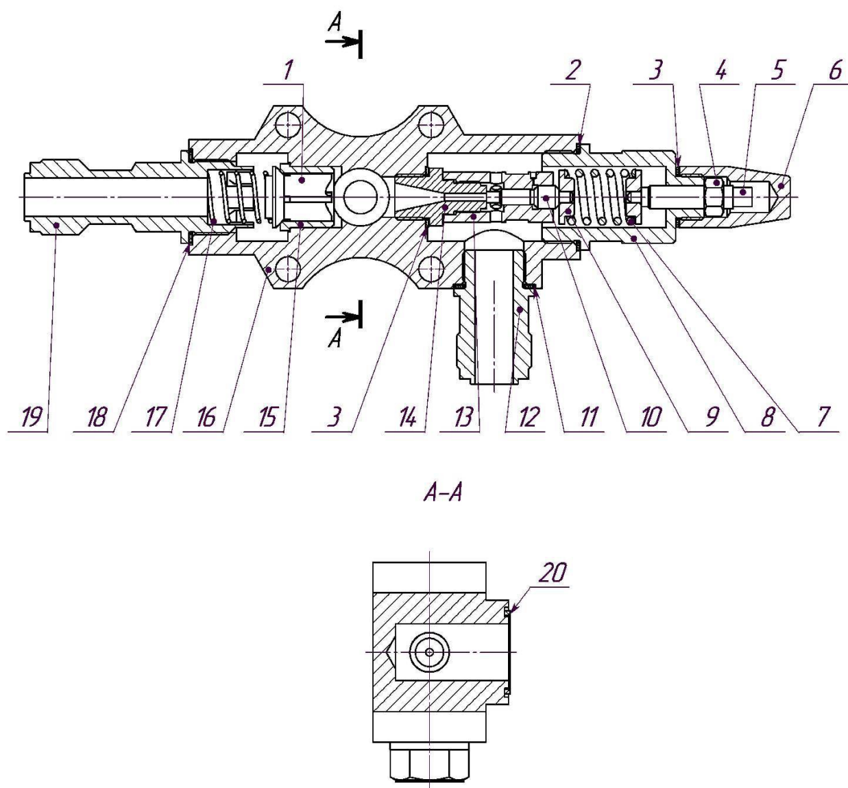
Рисунок 3 – Блок клапанный
