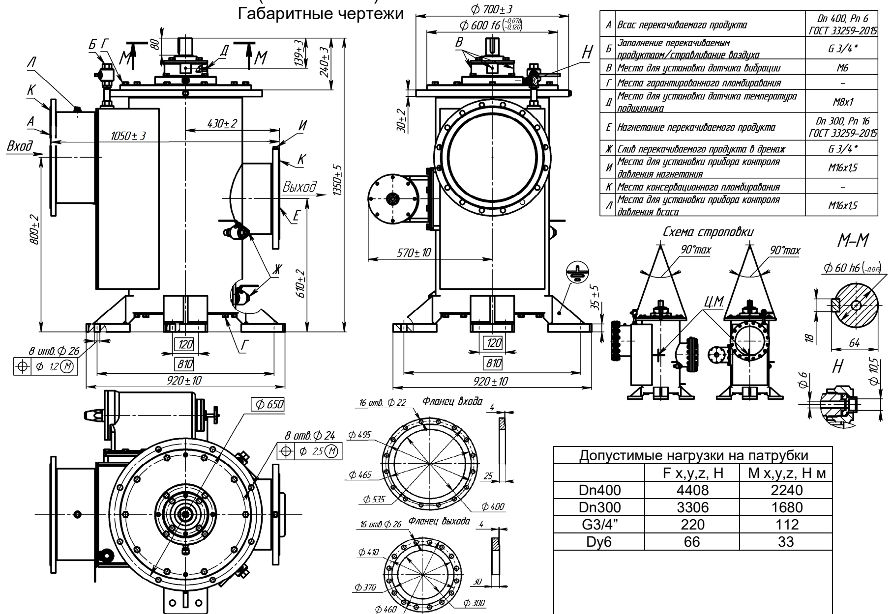
Рисунок Б.1 – Габаритный чертеж насоса А1 3Вх2 630/105
