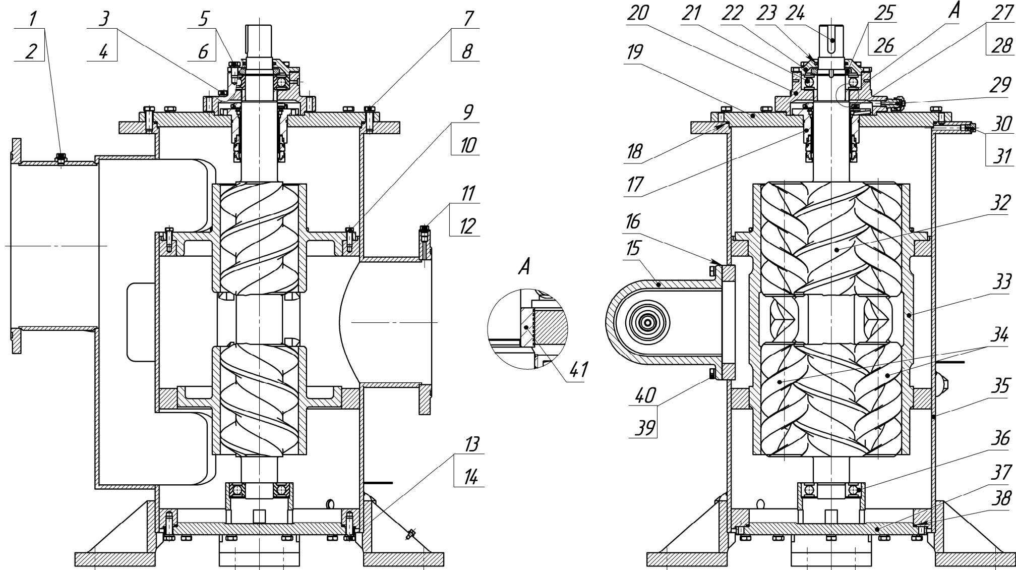
Рисунок 1 – Устройство насоса
