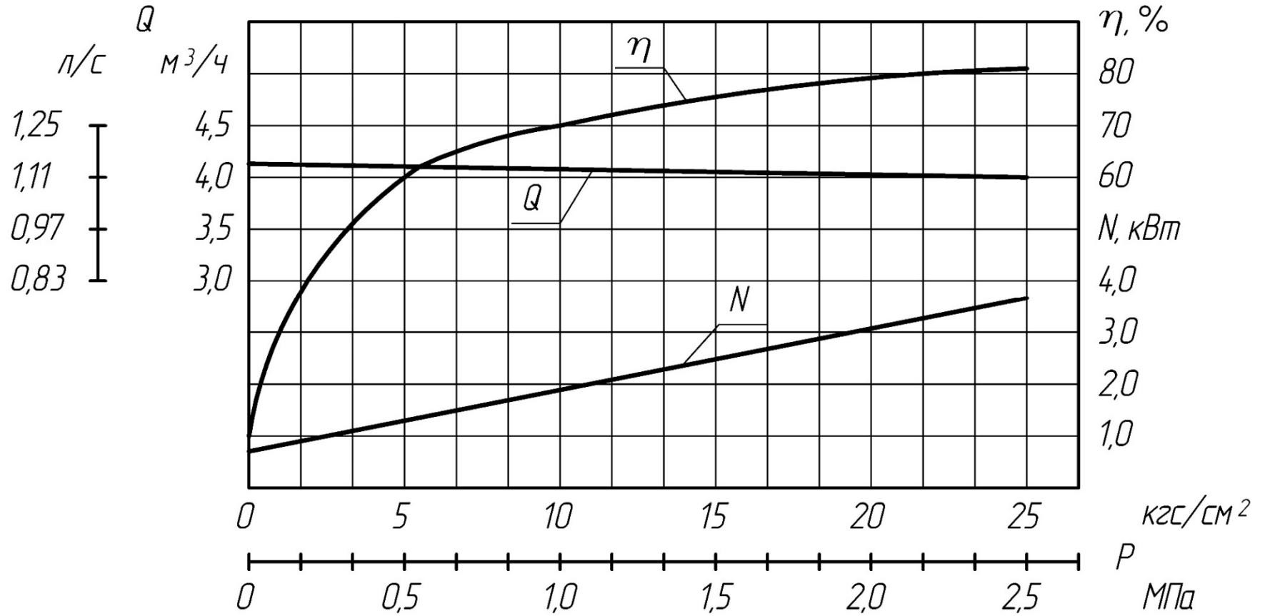
Рисунок В.2 - Характеристики насосов и агрегатов НМШ 5-25-4,0/4, НМШ 5-25-4,0/10, НМШ 5-25-4,0/25
