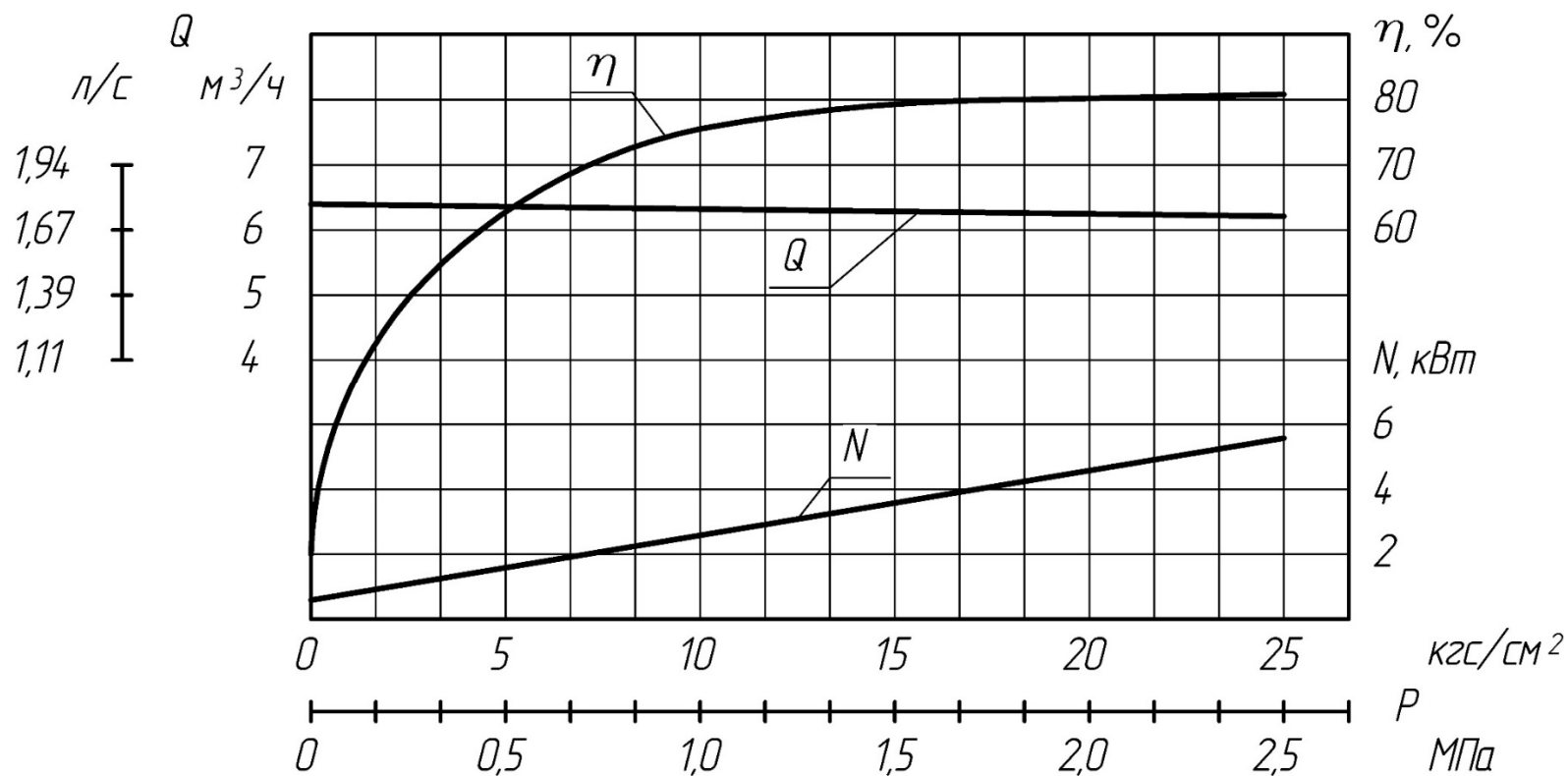
Рисунок В.4- Характеристики насосов и агрегатов НМШ 8-25-6,3/2,5, НМШ 8-25-6,3/4, НМШ 8-25-6,3/6, НМШ 8-25-6,3/10, НМШ 8-25-6,3/25
