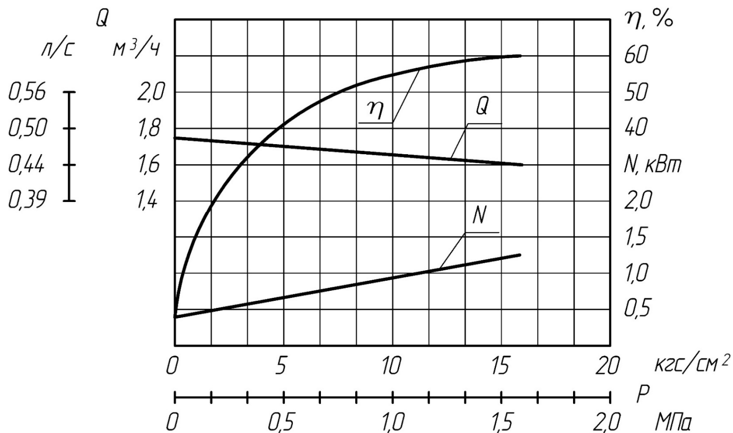
Рисунок В.1 - Характеристики насосов и агрегатов НМШ 2-25-1,6/4, НМШ 2-25-1,6/6, НМШ 2-25-1,6/10, НМШ 2-25-1,6/16
