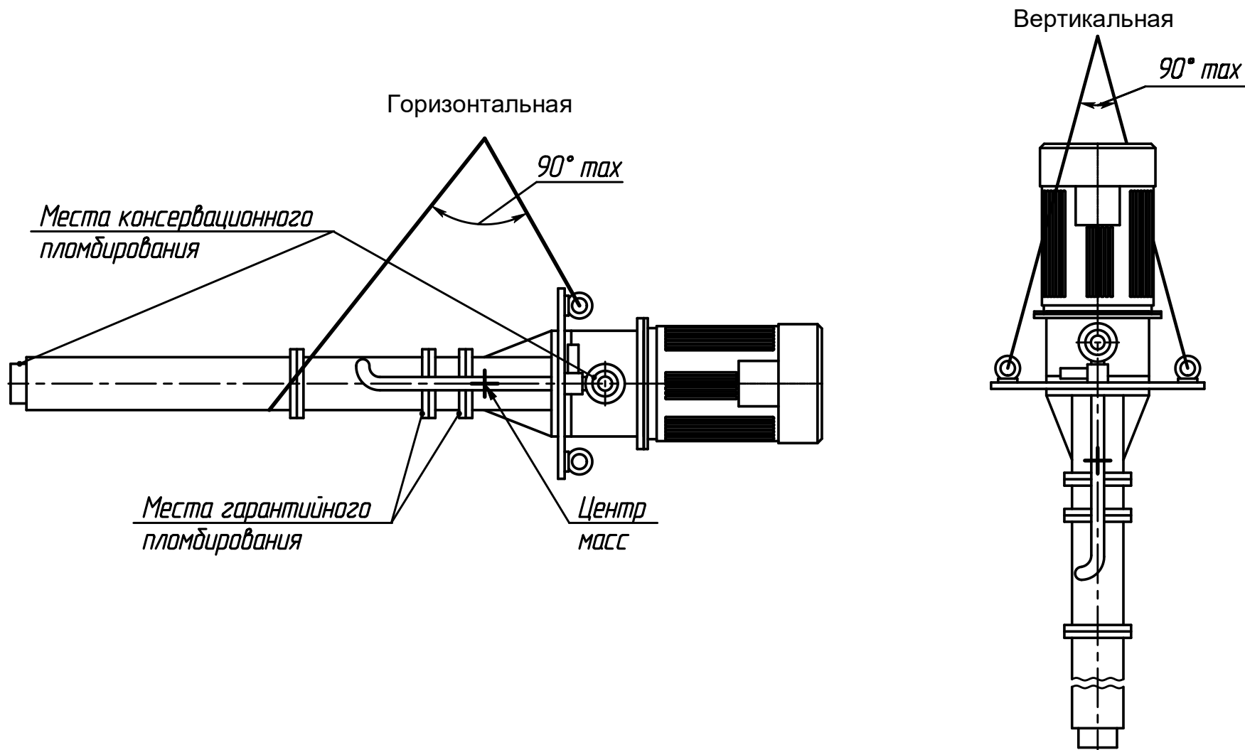
Рисунок В.1 – Схема строповки агрегатов
