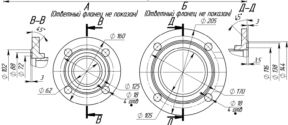
Рисунок Б.2 - Габаритный чертеж насоса А3 3В 16/25
