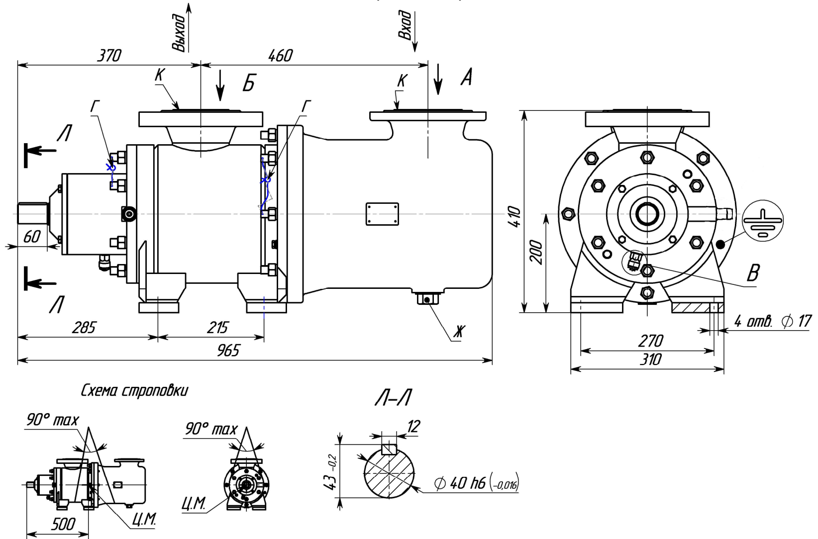
Рисунок Б.1 – Габаритный чертеж насоса А1 3В 63/40
