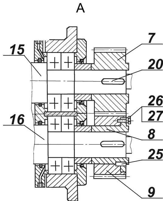
Рисунок Г.1 - Ремонтный комплект для насосов типа А5 2ВВ
