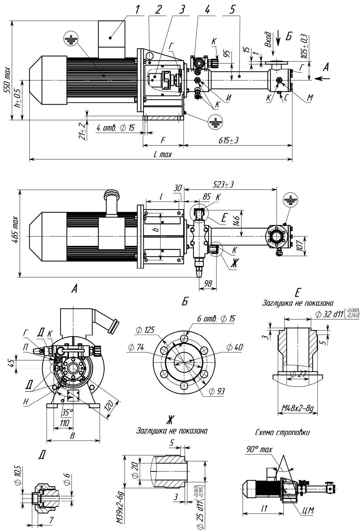
Рисунок Б.2 – Габаритный чертеж агрегата
