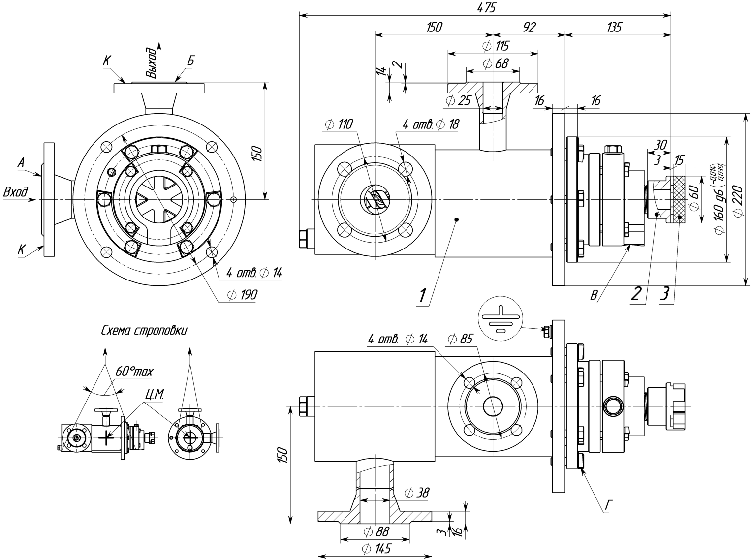
Рисунок Б.1 – Габаритный чертеж насосов А1 3В 3/16, А3 3В 3/16
