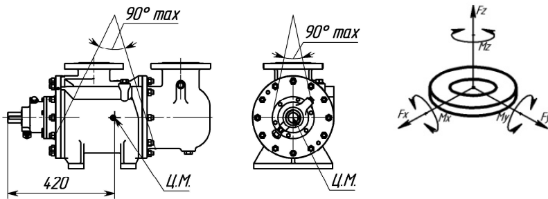
Схема строповки
