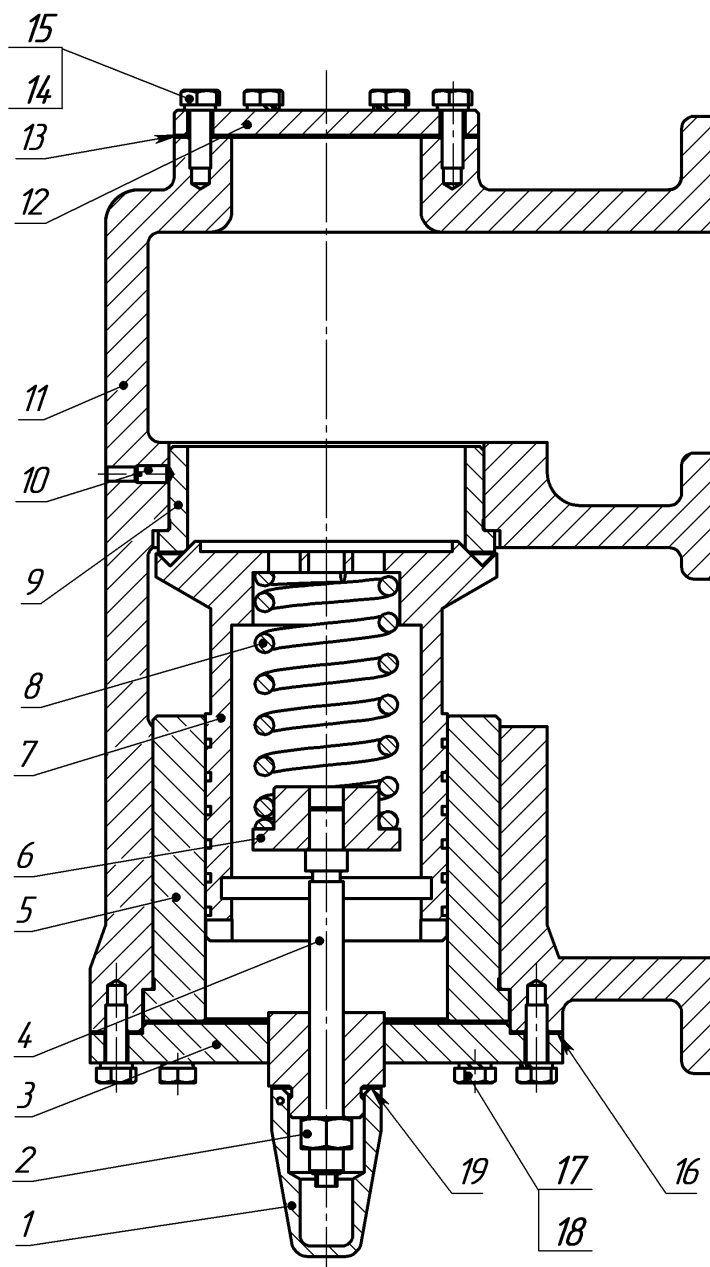
Рисунок 2 – Клапан предохранительный
