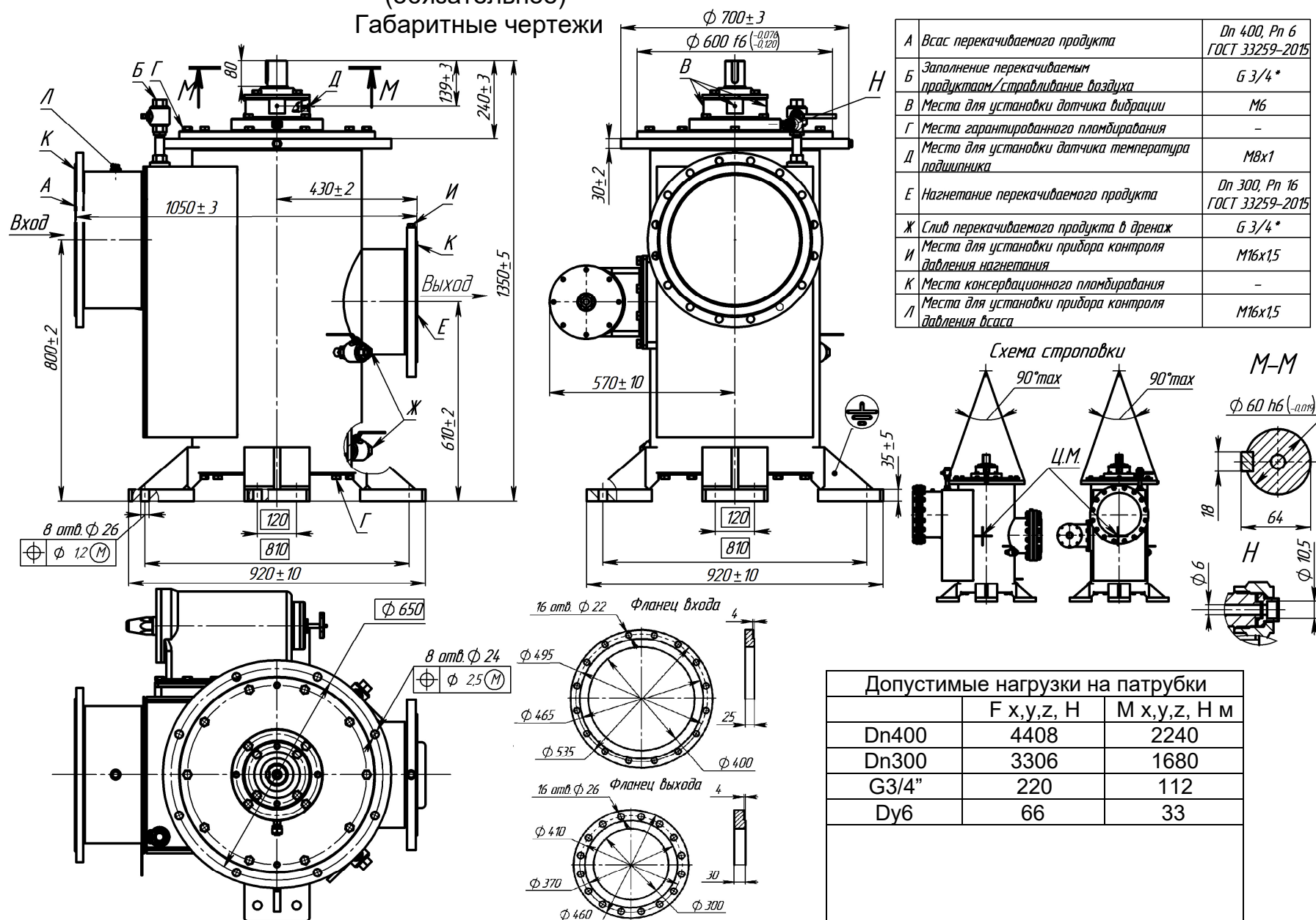
Рисунок Б.1 – Габаритный чертеж насоса А1 3Вх2 630/10Б
