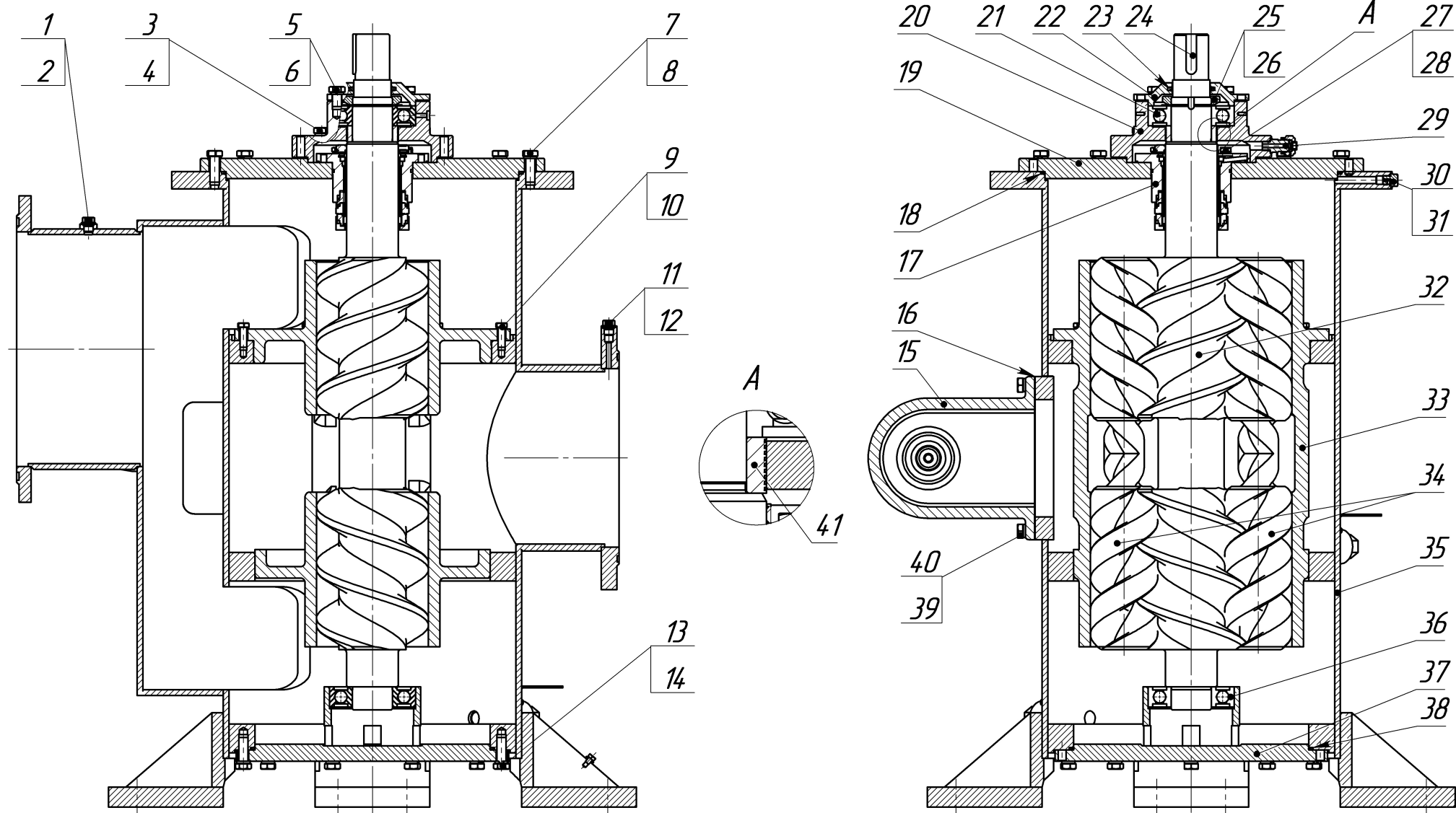
Рисунок 1 – Устройство насоса
