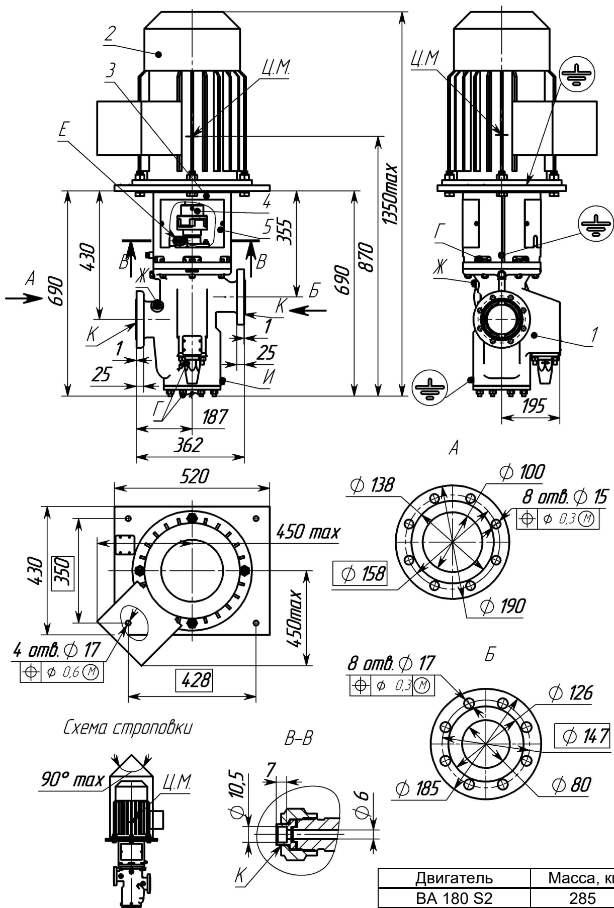
Рисунок Б.2 – Габаритный чертеж электронасосного агрегата
