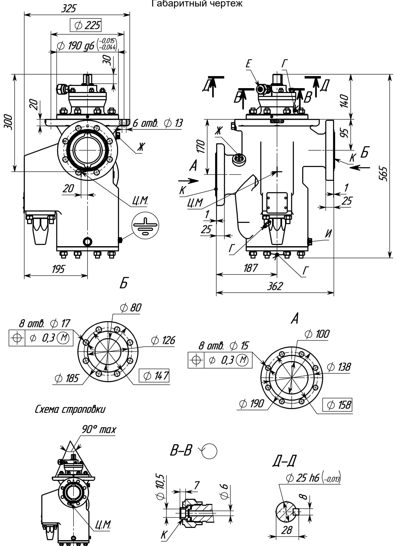
Рисунок Б.1 – Габаритный чертеж насоса
