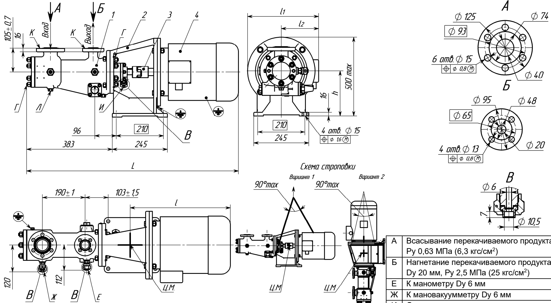
Рисунок Б.2 – Габаритный чертеж агрегата
